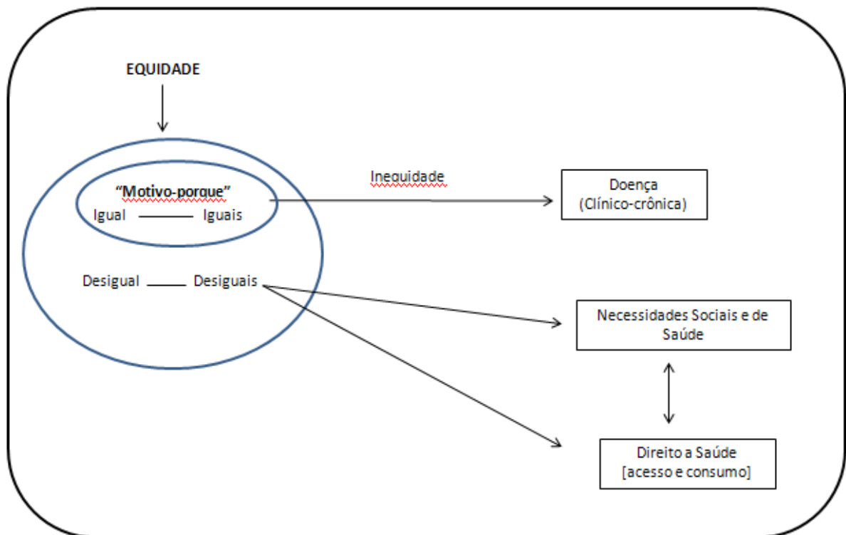
Figura 4 – Saúde como Direito e Equidade
