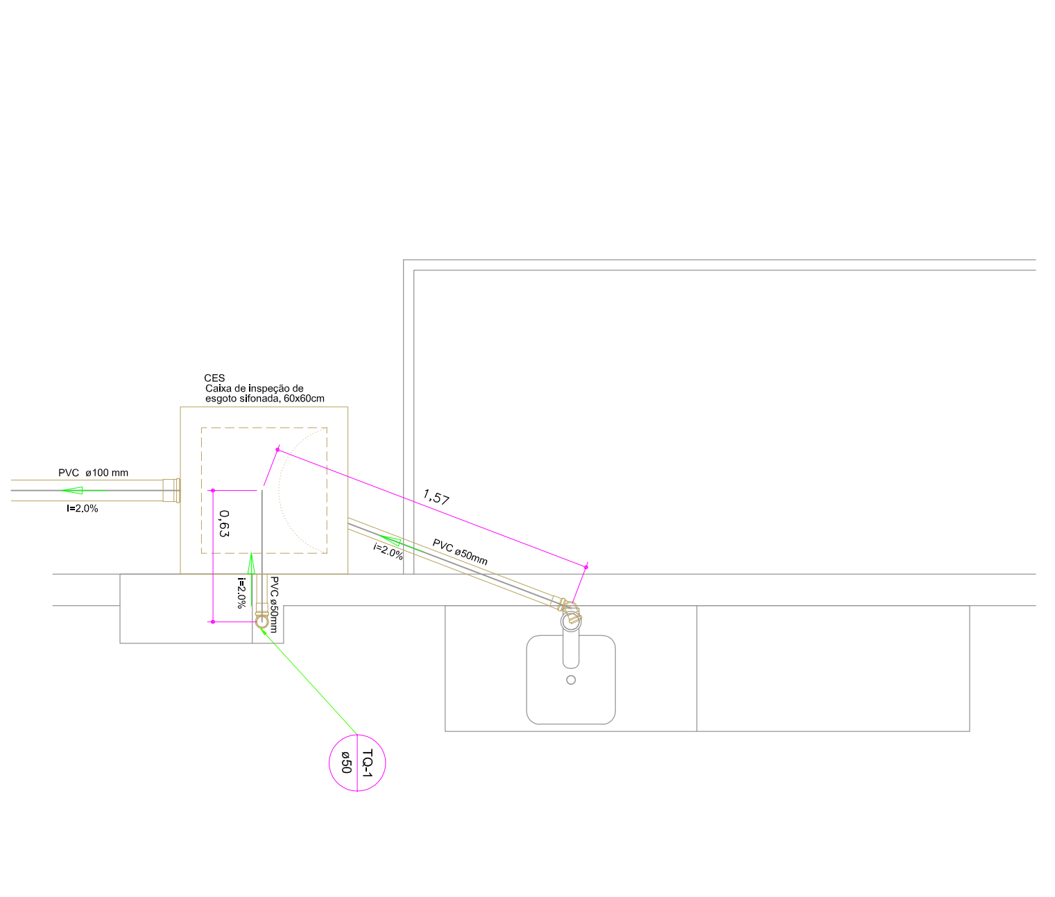
2 ESC 125 DETALHE S7/S8/S9/DEPOSITO DO SALÃO DE EXPOSIÇÃO - 1º PAVIMENTO/ÁREA B
